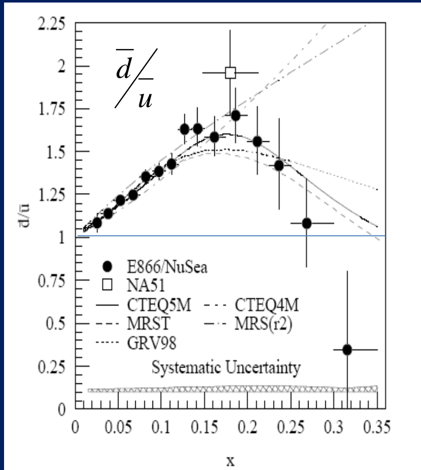
E866: PRD64, 052002 (2001)
