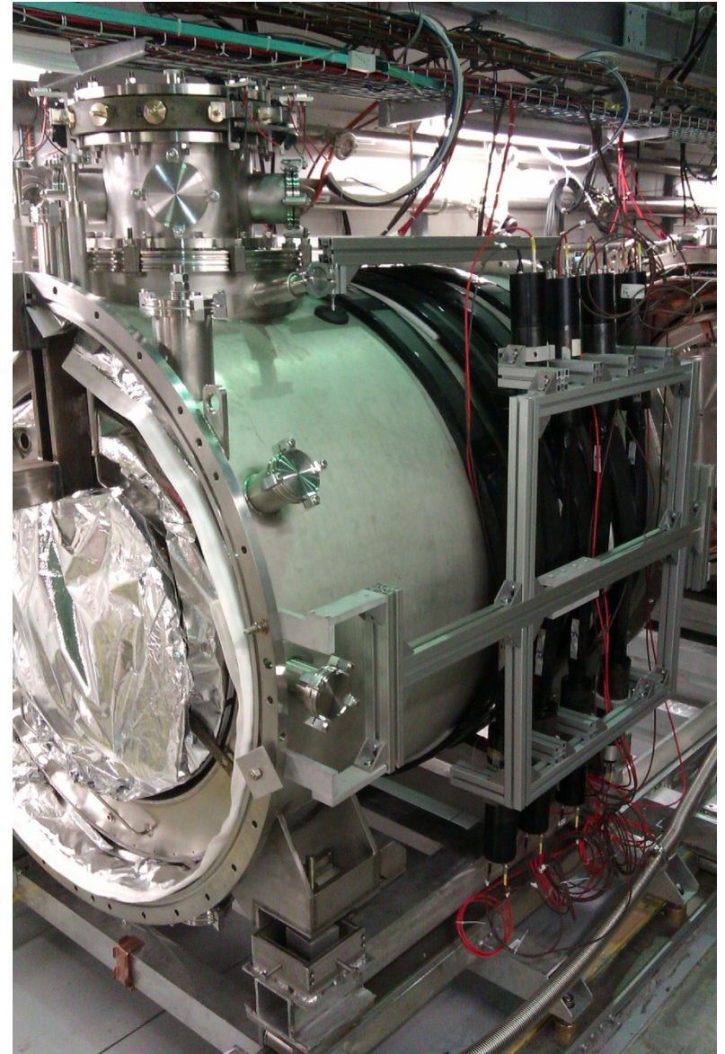
Criostato 1T
