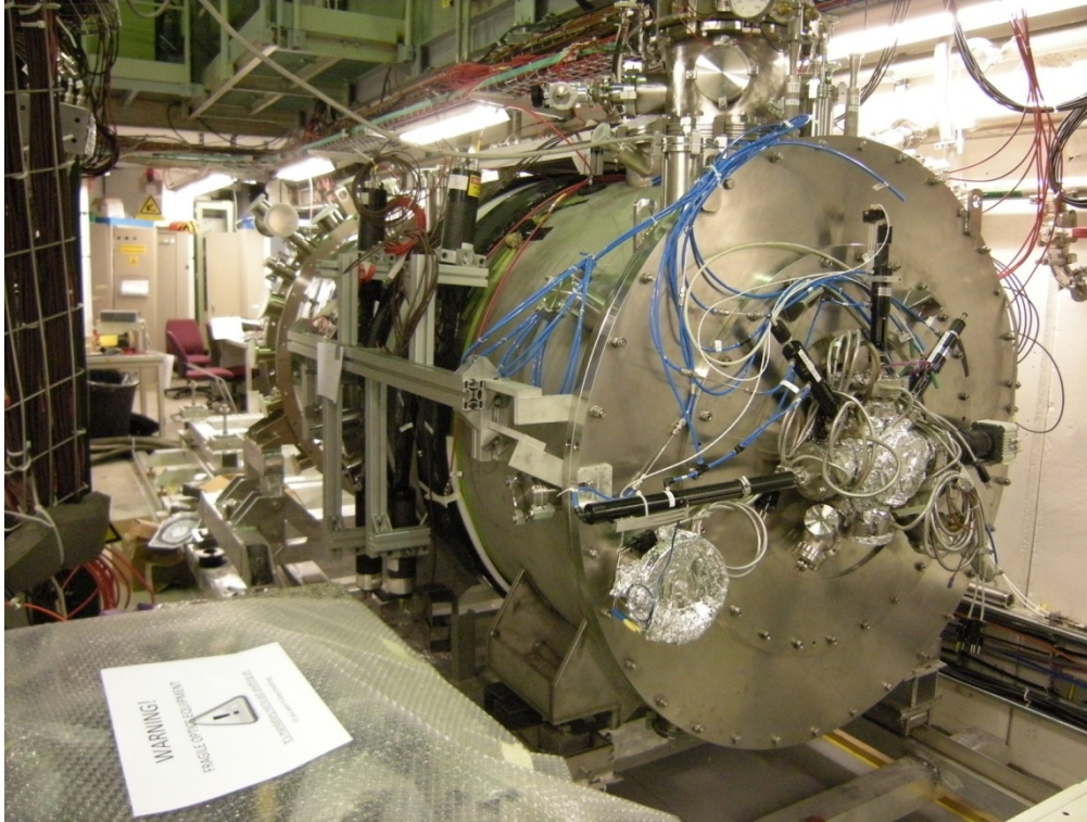
Criostato 5T
