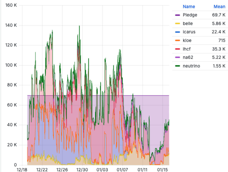
HEPScore usage Gruppo 1
