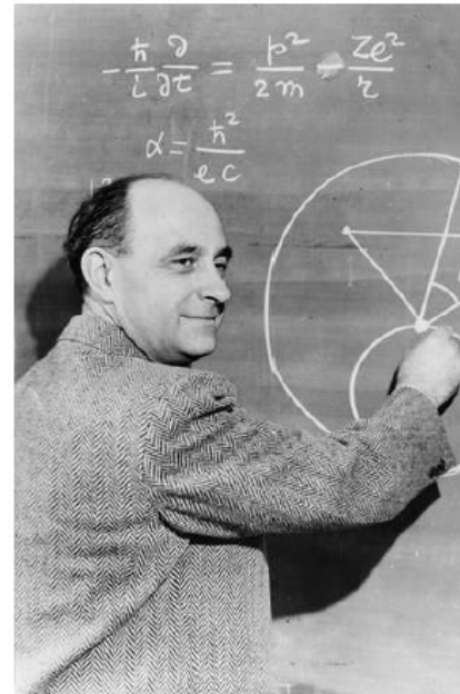
Enrico Fermi
