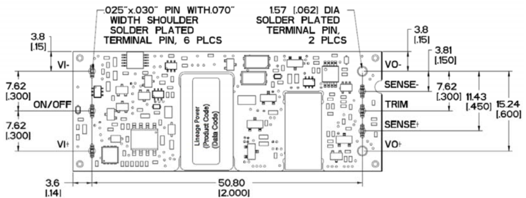
Bottom View#
