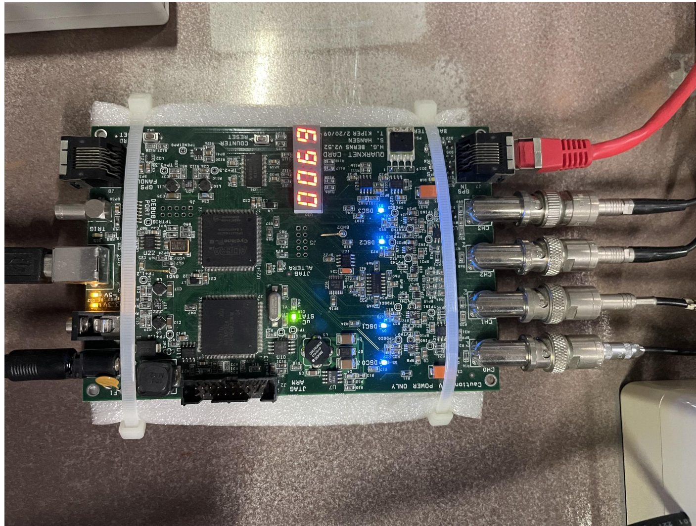
La scheda di front-end per le coincidenze
