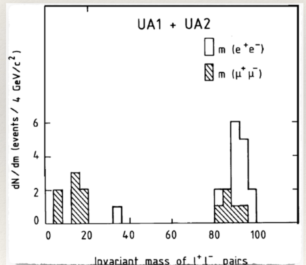
Plot di scoperta del bosone Z nel 1983
