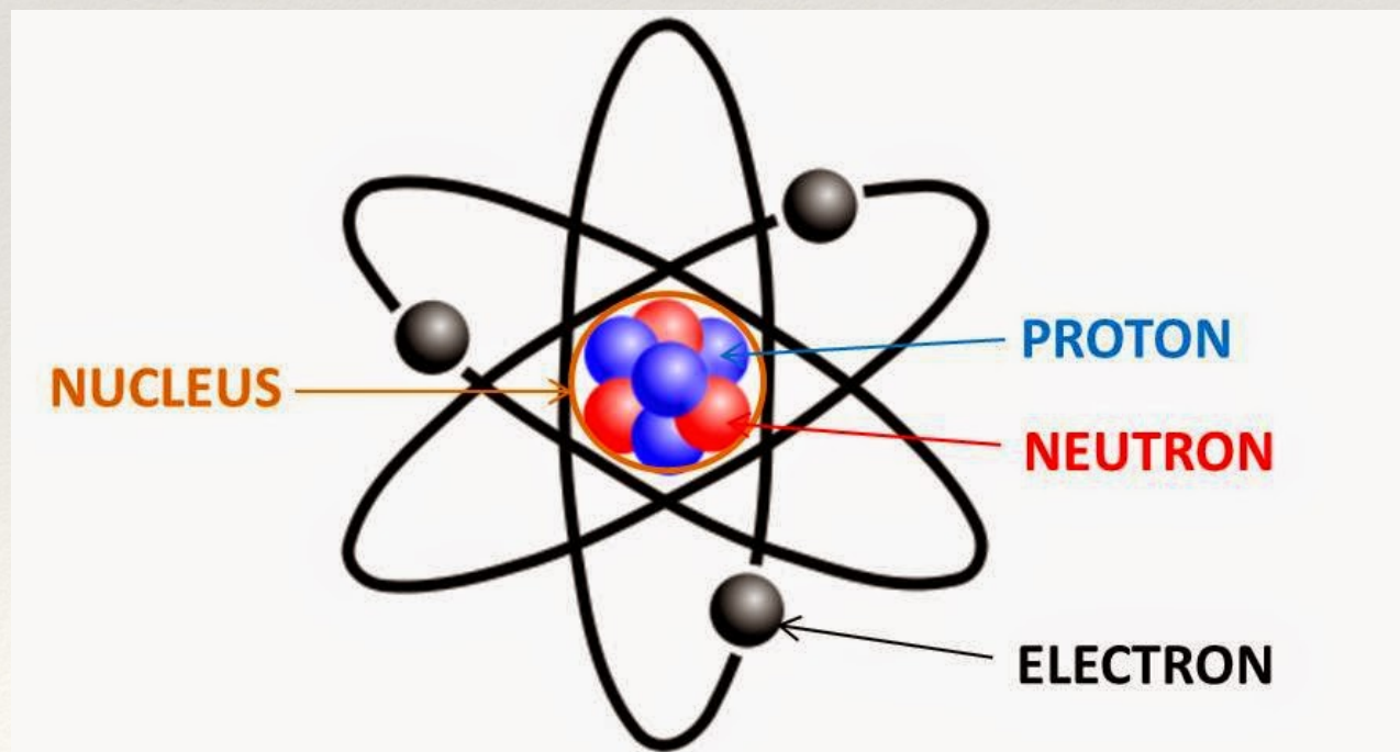
Atomo
