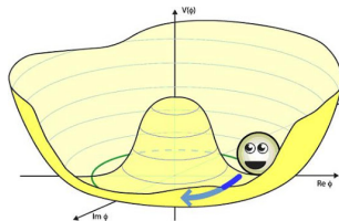
fase stabile (vuoto), non simmetrica
