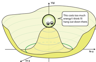
fase simmetrica, non stabile
