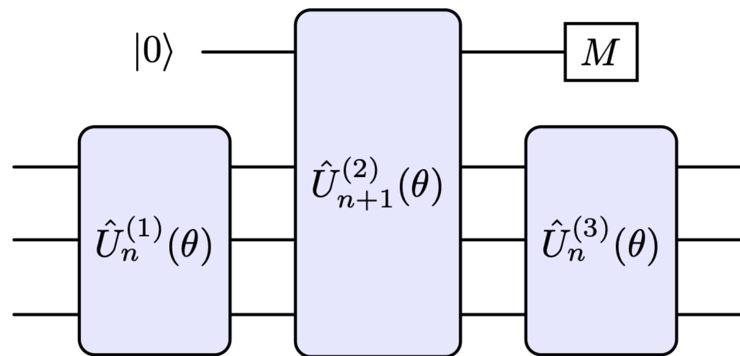
Quantum hardware-oriented ansatz
