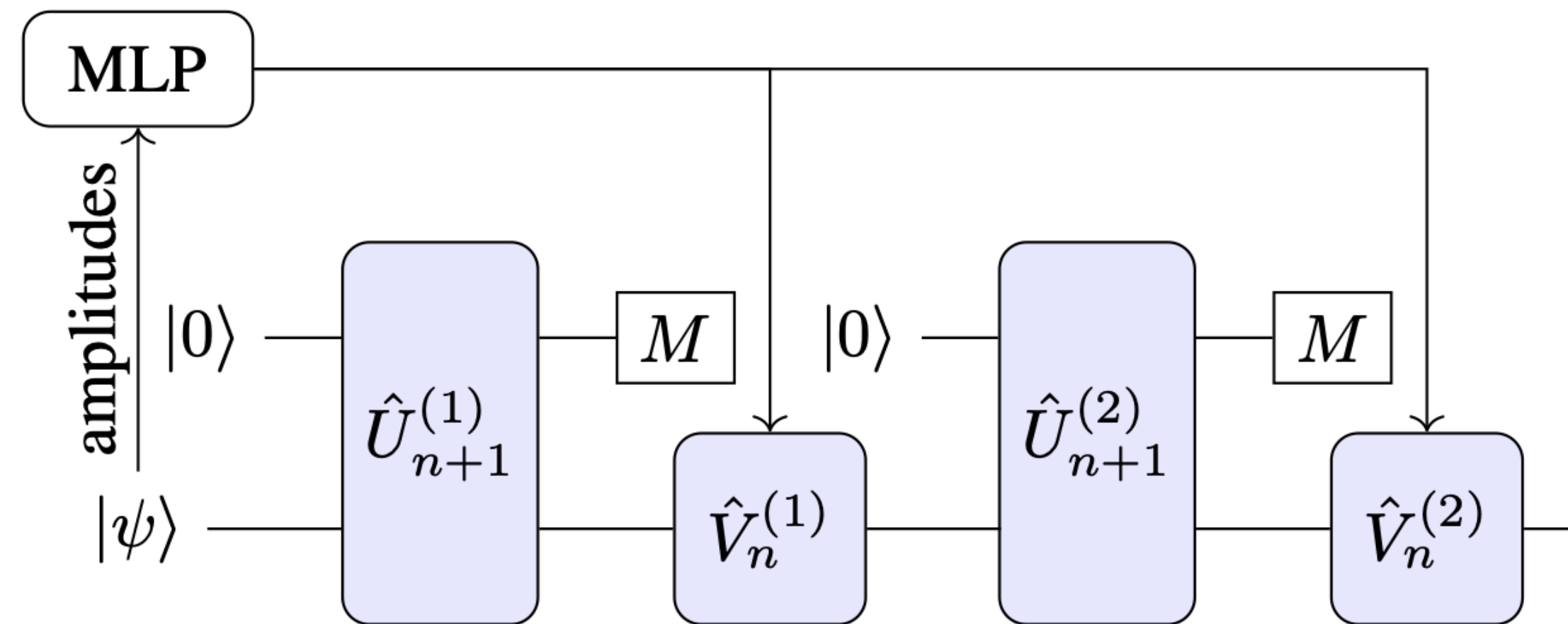
Hybrid ansatz (NN + PQC)
