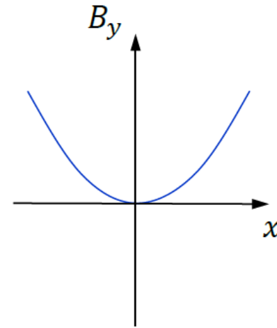
B_3 : sextupole
