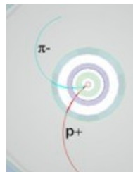
\Lambda \rightarrow p \pi^-
