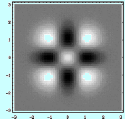
TEM_{22}
