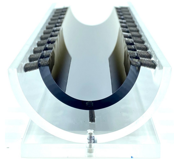
2026: un rivelatore 'trasparente'
