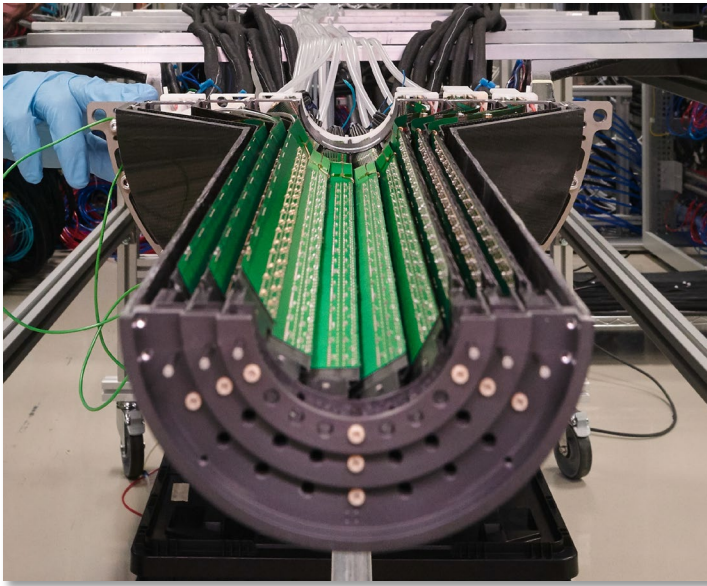
2021: un rivelatore leggero
