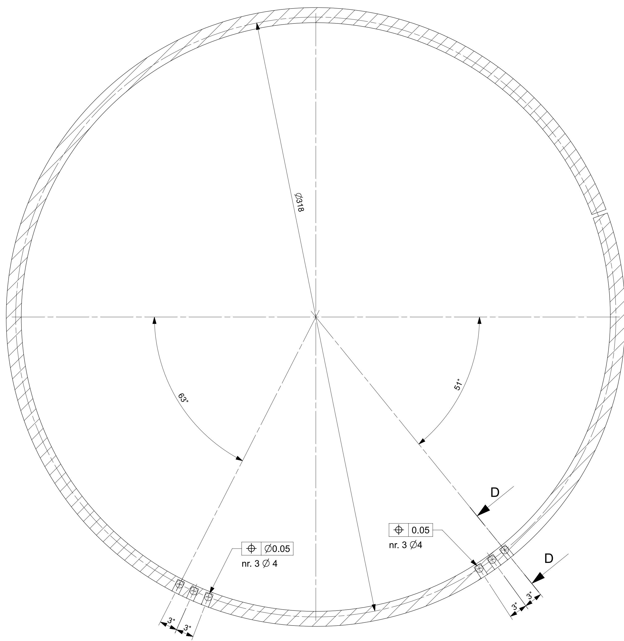
SECTION A-A
