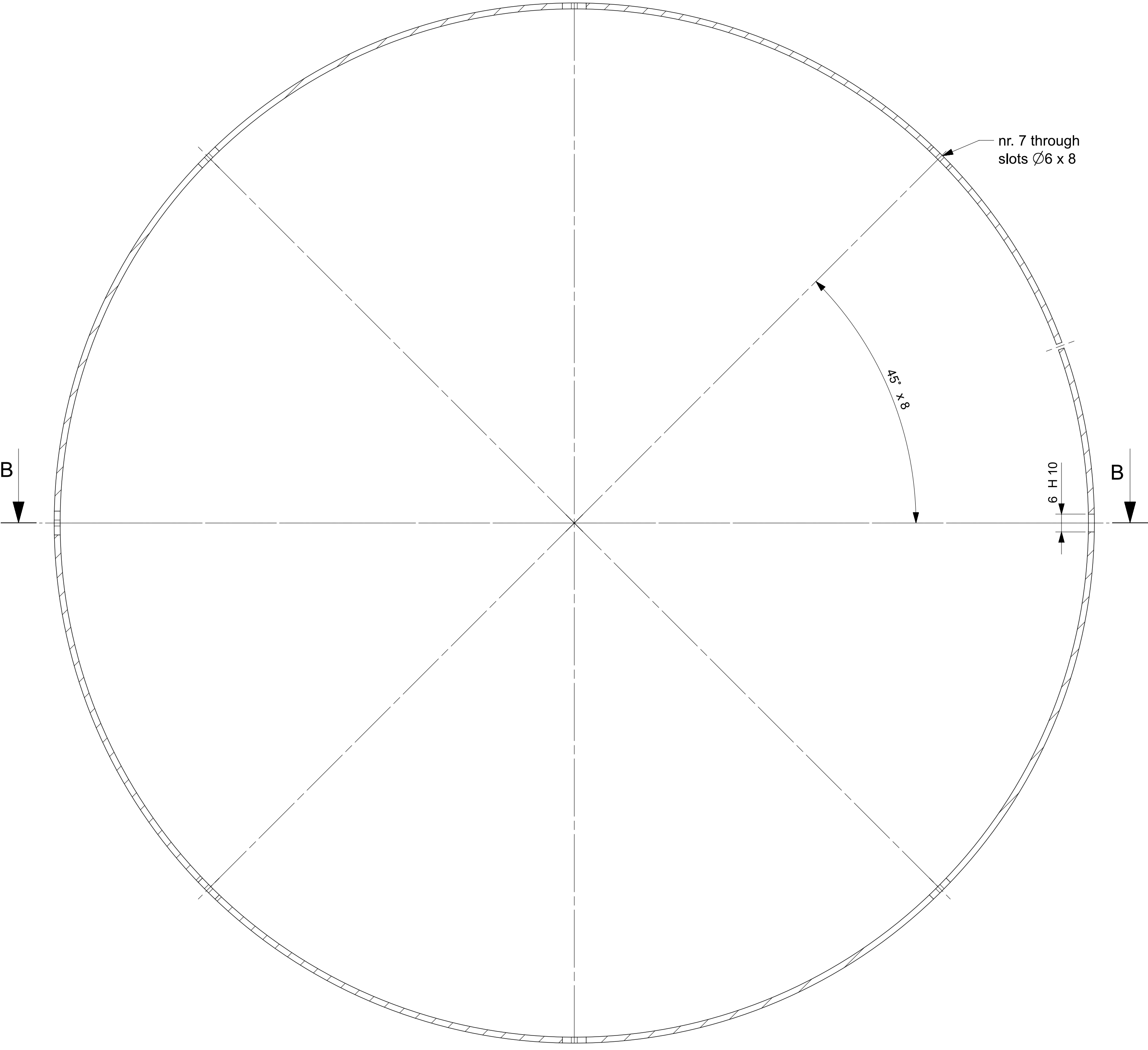
SECTION A-A
