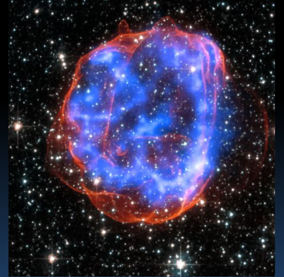
Resti di supernove
