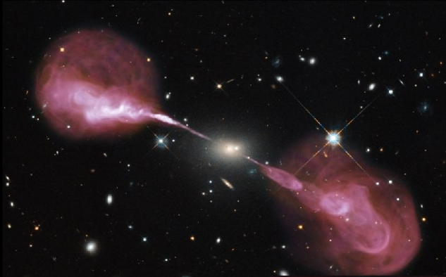
Hercules A radio jets
