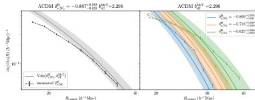
Voids abundance
