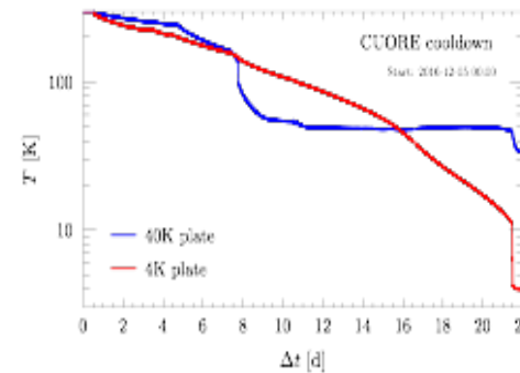
Cooldown 300 \rightarrow 4K
