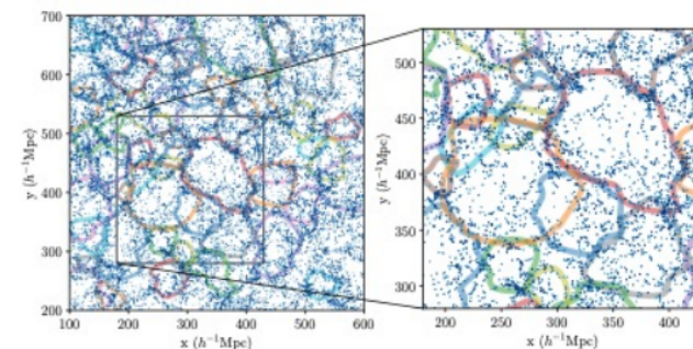
Voids abundance
