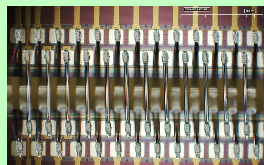
wire bonds
