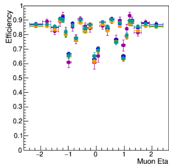
WHOLE DETECTOR, Eta dependence
