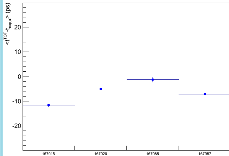
t-t_{\text{exp}} (gaussian fit)
