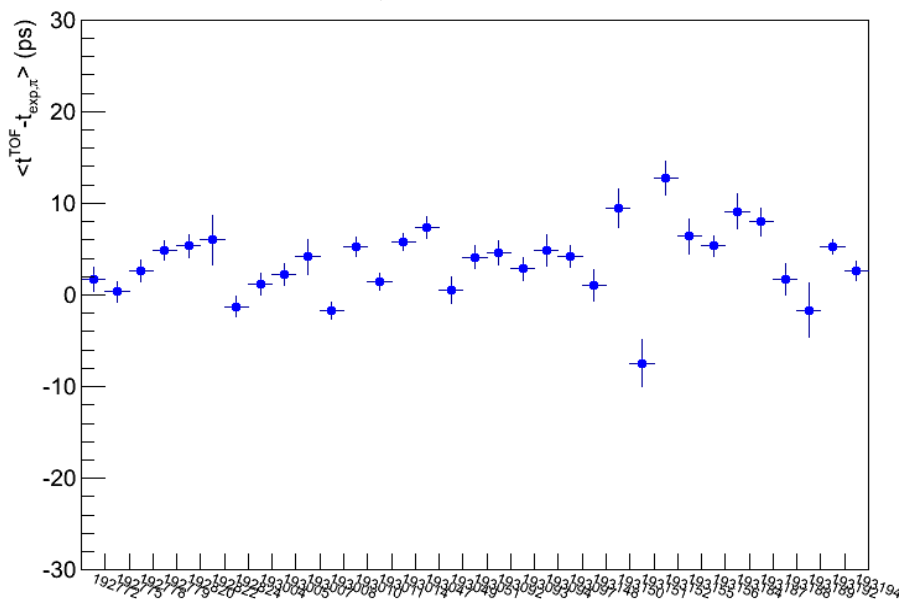
t-t_{\text{exp}} (gaussian fit)
